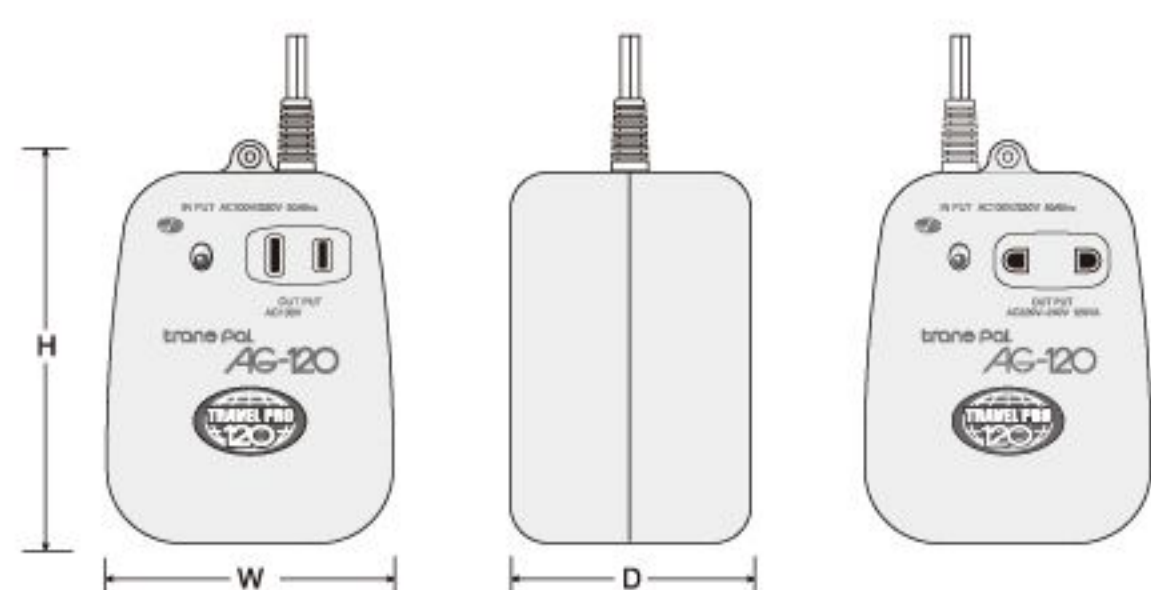
形状・寸法図 AG-120
