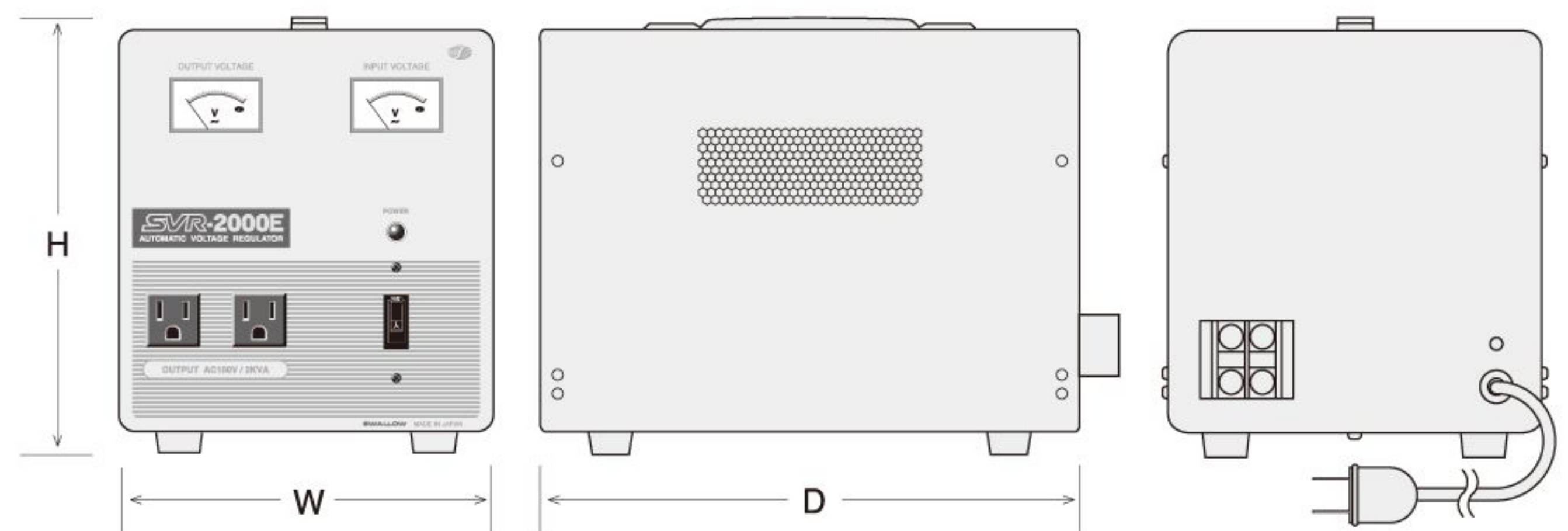
AVR-2000E
