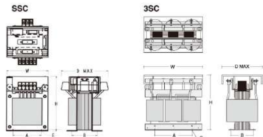
形状・寸法図
